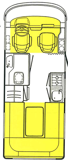
L-Sitzgruppe Variante im 660 auf Wunsch.
