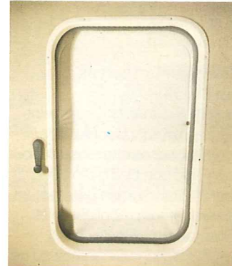
Großvolumiger, stufenlos verstellbarer und weit überragender Eriba-Hymer-Kurbeldachlüfter mit integrierter Isolationsmatte.
